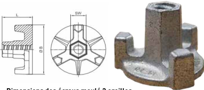
Dimensions des écrous moulé 3 oreilles
