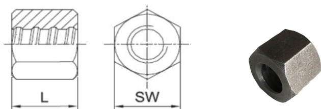
Dimensions des contre écrous hexagonaux (finition brut)
