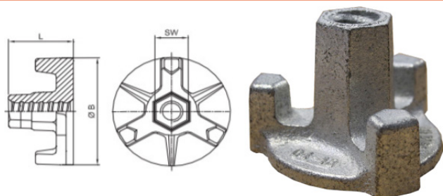
Dimensions des écrous moulés 3 oreilles
