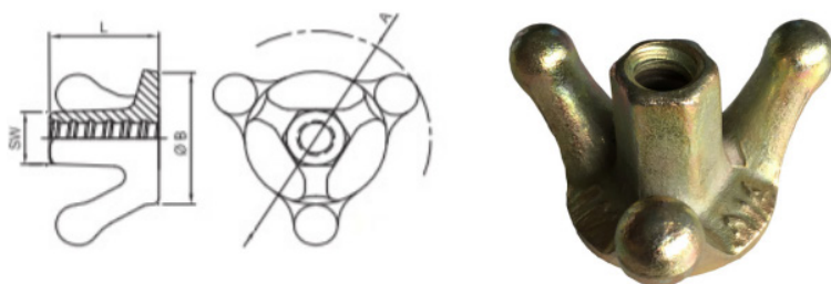
Dimensions des écrous forgés 3 oreilles
