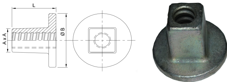
Dimensions des écrous base carré SATECO
