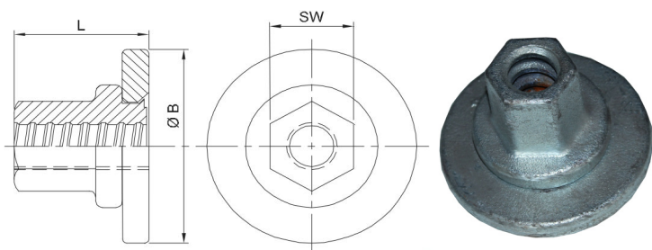
Dimensions des écrous base flottante SATECO
