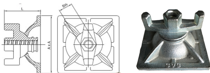
Dimensions des écrous moulés 2 ailettes rotatif
