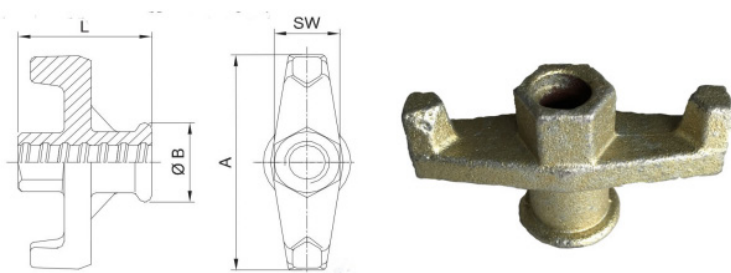
Dimensions des écrous moulés 2 oreilles
