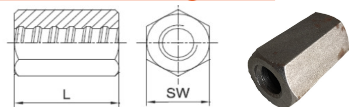
Dimensions des contre écrous hexagonaux
