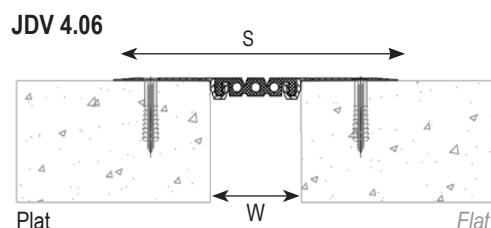
JDV 4.06 Cornières apparentes fixées mécaniquement Visible mechanically fixed aluminium side plates
