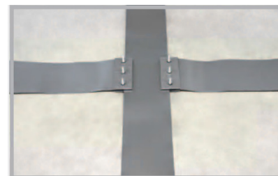
Raccord en croix
