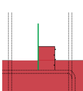
Phase 1 : Coulage du radier, le talon est rempli en même temps.
