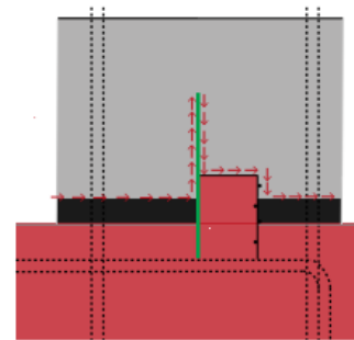
Cheminement de l'eau multiplié par 3.
