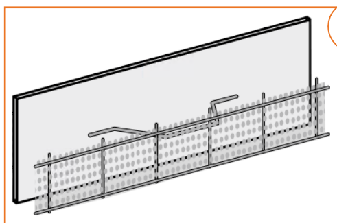
Avec tôle d'étanchéité simple
