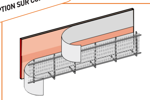
Avec tôle d'étanchéité enduite Butyle 50mm
