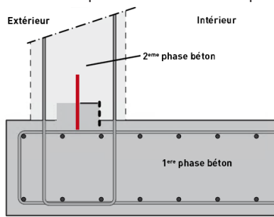
Modèle Simple
