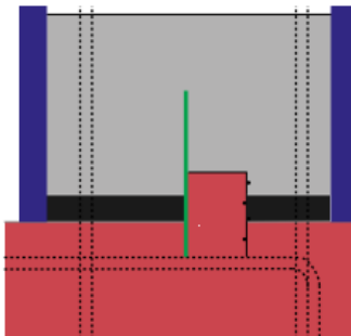
Phase 3 : Pose des banches facilitée par la talonette, avec un radier en pente la
