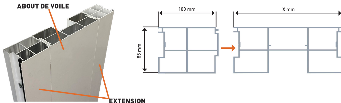
Dimensions des extensions about de voile
