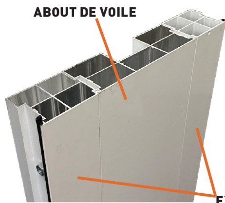
Dimensions des extensions about de voile
