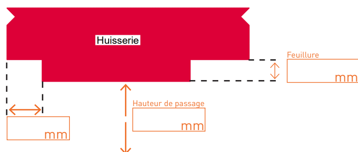
Coupe vericale
