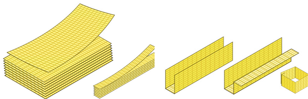
Coffrage pré-plié en forme de U
